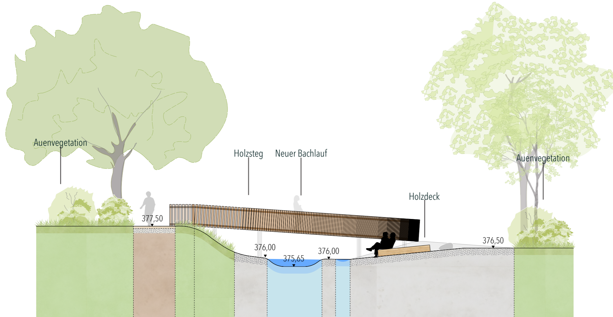
DETAILSCHNITT 01 | AUENBEREICH DES SCHILTERNBACHS MIT STEG
